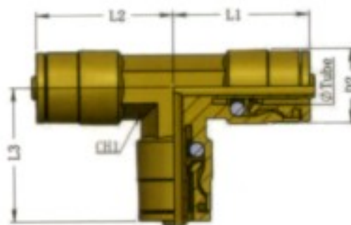
DOT-HUC 等径三通 CR-293
