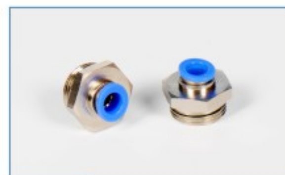
CR-105 M12x1.5 M14x1.5 M16x1.5 M18x1.5 M22x1.5 Ø6 Ø8 Ø10 Ø12 Ø15
