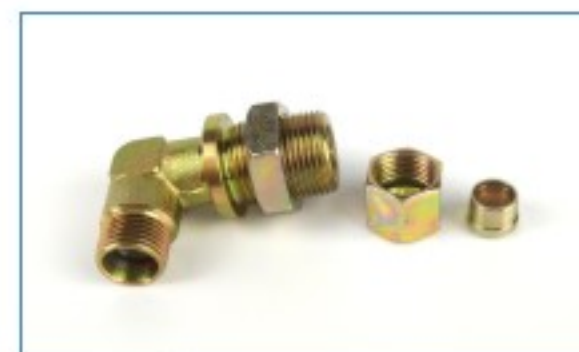
CR-021 M18x1.5-M22x1.5 M16x1.5-M22x1.5 M22x1.5-M22x1.5
