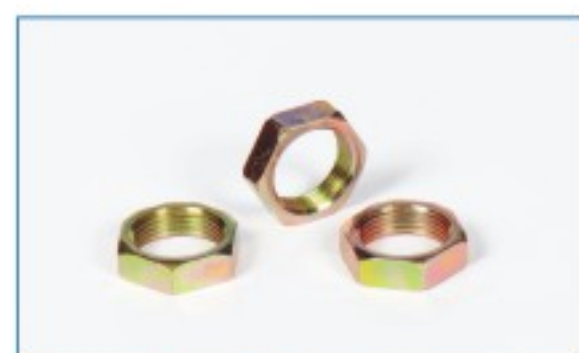
CR-015 M12x1.5 M14x1.5 M16x1.5 M18x1.5 M22x1.5
