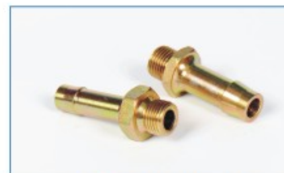
CR-024 M22x1.5-Ø16 M16x1.5-Ø13 M16x1.5-Ø11
